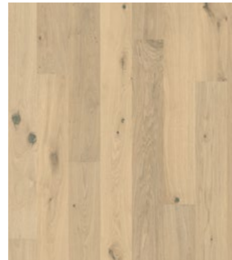
Eiche Edelweiß 2266 ×187×13 mm 3-Schicht, Nutzschrift ca 2,5 mm, naturgeölt 77003208
